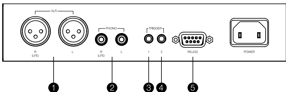
Diagrama 3 Panel de conexiones del subwoofer DB
